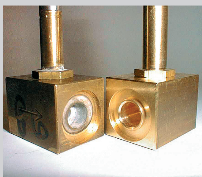
Corrosión de partes mecánicas al utilizar un aditivo incorrecto o agresivo o alcohol de baja calidad. Foto: Technotrans.
