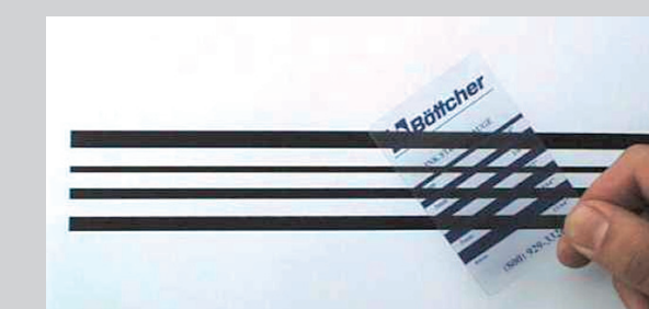
Asegurar siempre que la franja de contacto es uniforme en toda la anchura de la máquina y comprobar los ajustes mediante una galga con franjas preimpresas. Foto: Böttcher.
