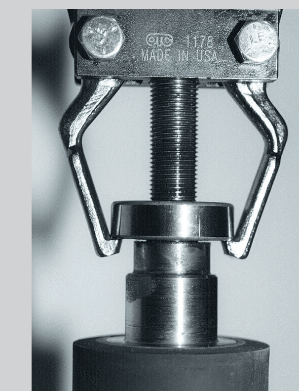
Utilizar siempre los utensilios adecuados para asegurar una colocación ajustada y recta de los cojinetes. Foto: Böttcher.
